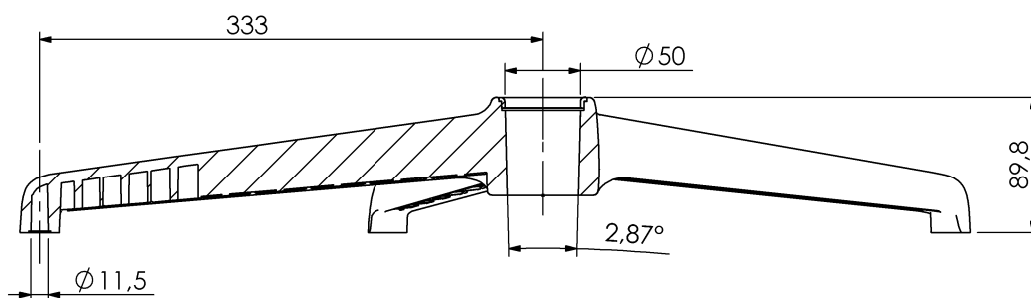
SEZIONE A-A SCALA 1 : 5
