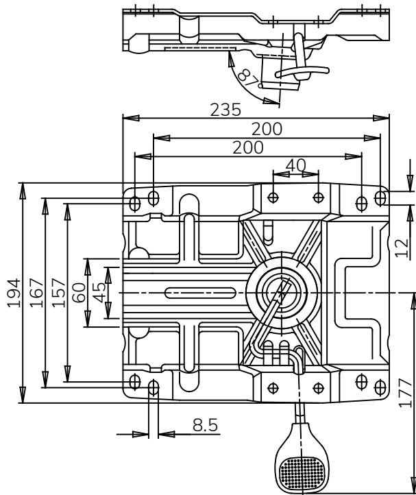
Piastra 961M4
