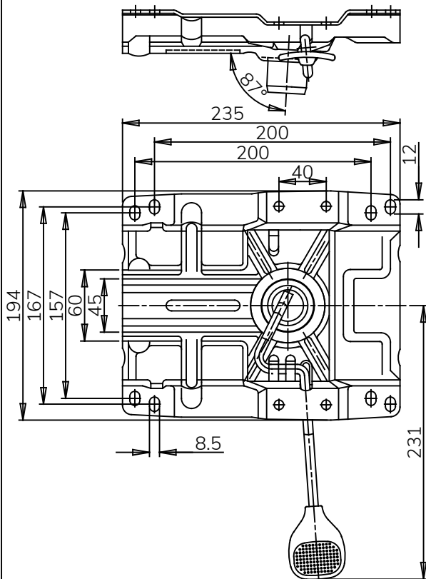
Piastra 961M4
