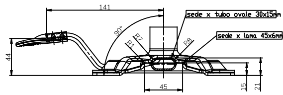
SEZIONE A - A
