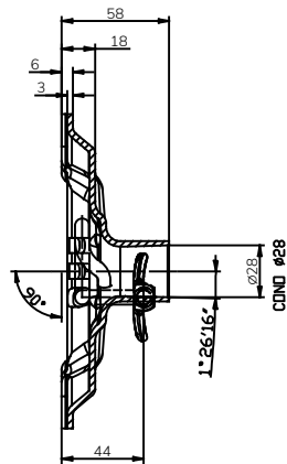
SEZIONE C - C
