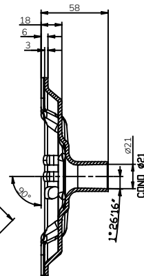
SEZIONE B - B
